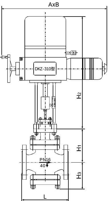
外形尺寸 单位: mm
