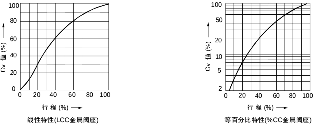
图1 流量特性曲线
