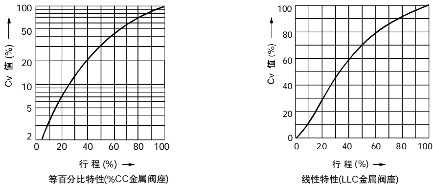
图1 流量特性曲线
