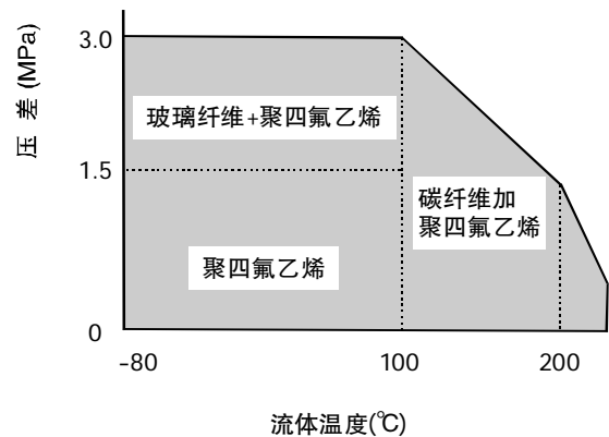
图2 软阀座的工作温度和压差的范围
