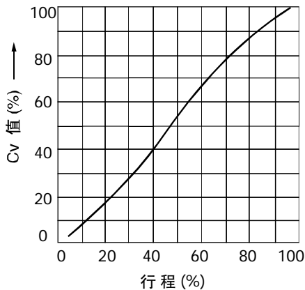
图1 流量特性曲线(线性LV)
