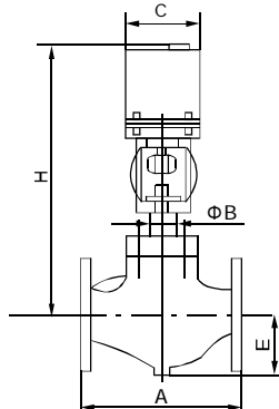
配361L执行机构电动阀外形图
