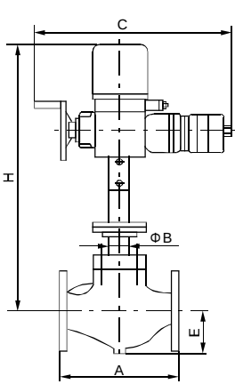
配DKZ执行机构电动阀外形图
