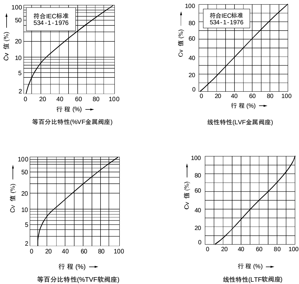
图1 高精度套筒的流量特性曲线
