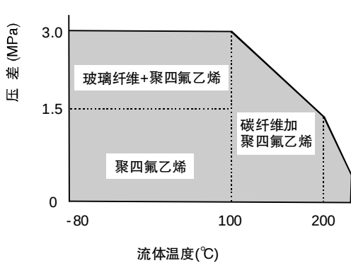
图3 软阀座的工作温度和压差的范围
