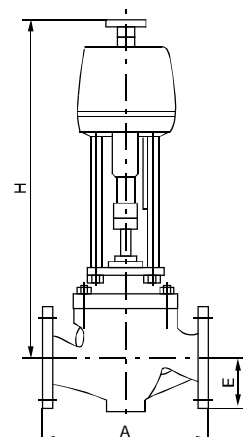
配PSL执行机构电动阀外形图
