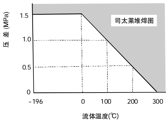
图3 需要堆焊司太莱合金的温度，常用压差范围。
