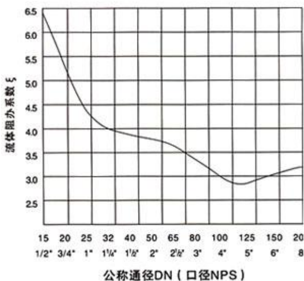
流体力学性能 H71对夹升降式止回阀的流体阻力径系数
